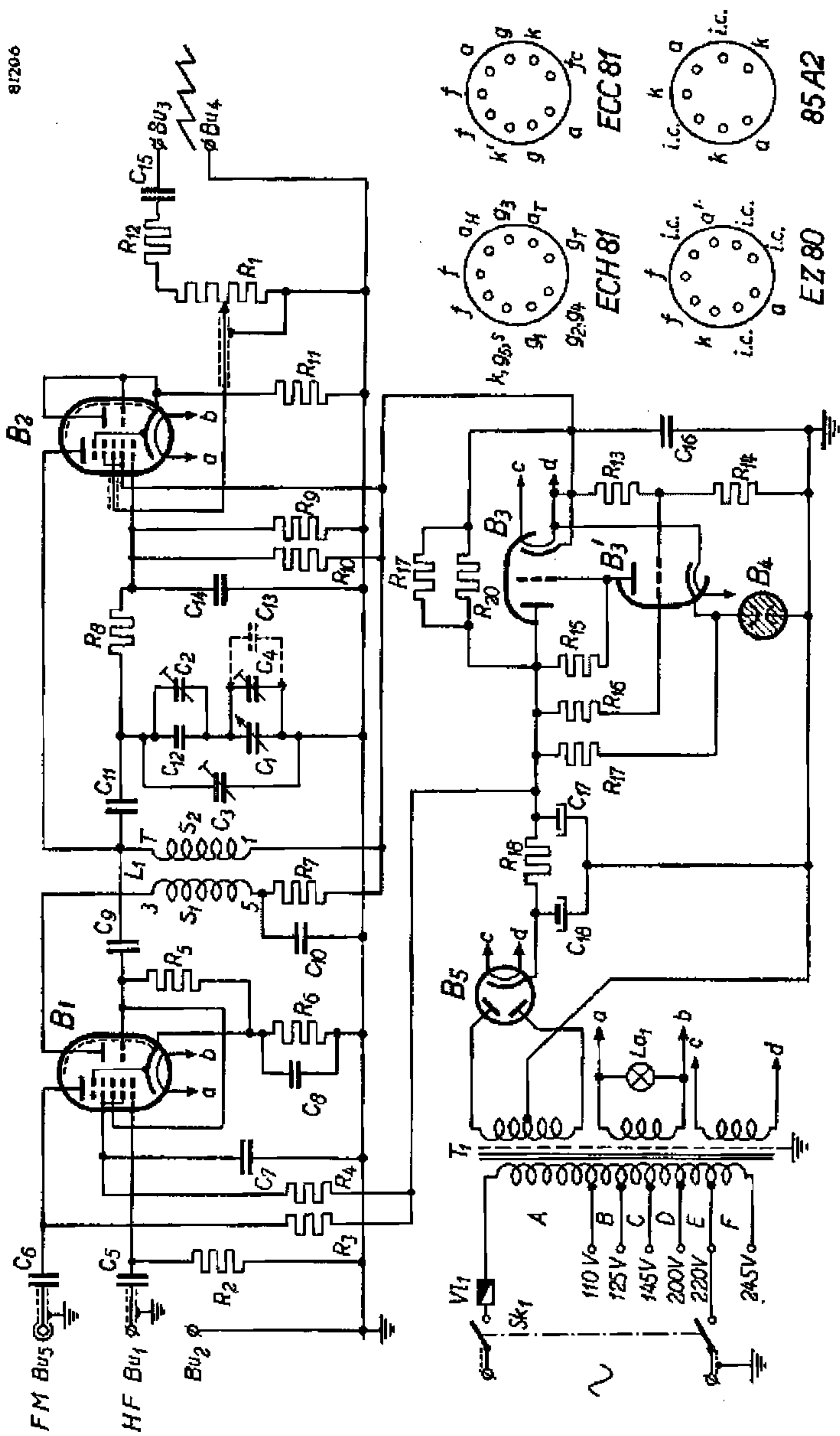
Fig. 8. Principeschema GM 2886/01 (geringe wijzigingen voorbehouden)
